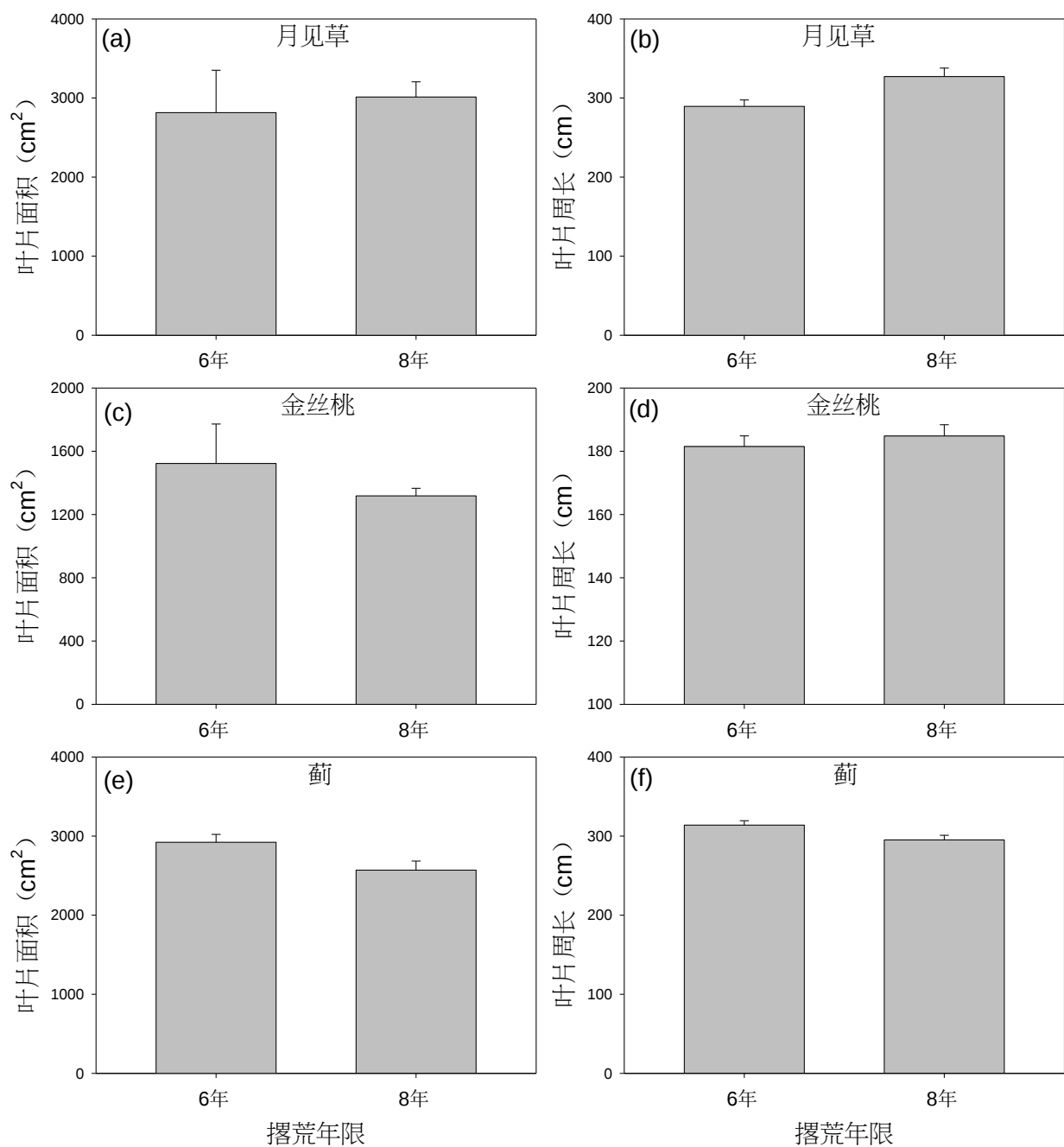
图 2 不同撂荒年限对月见草、金丝桃和蓟的叶片面积和周长的影响
