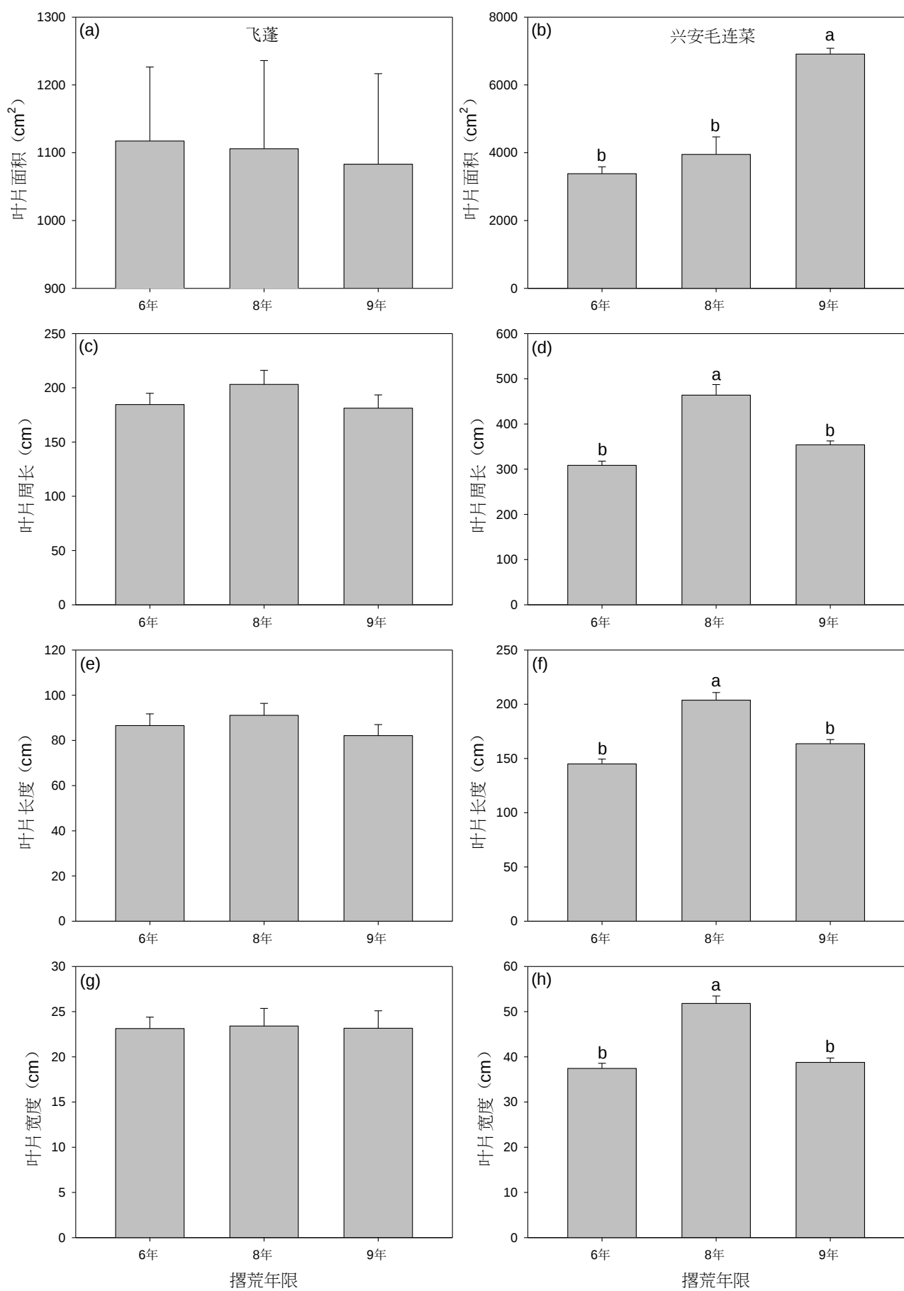
图 1 不同撂荒年限对飞蓬和兴安毛连菜叶片面积、周长、长度和宽度的影响
