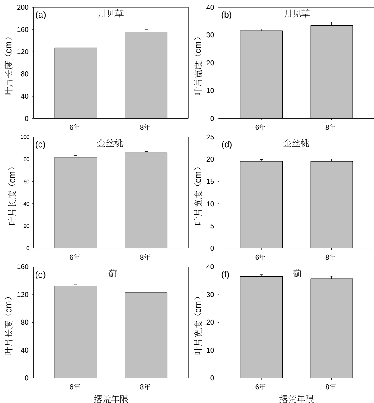
图 3 不同撿荒年限对月见草、金丝桃和蓟的叶片长度和宽度的影响
